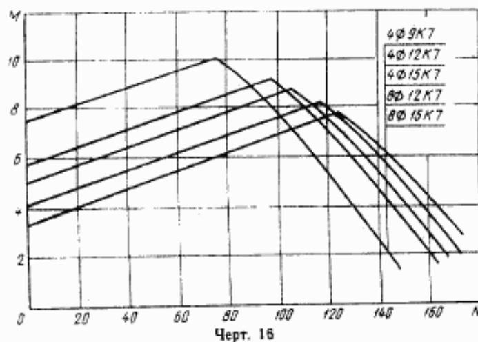
Сваи сечением 35×35 см. Бетон М400
